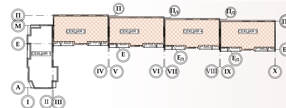
СХЕМА БЛОКИРОВКИ
